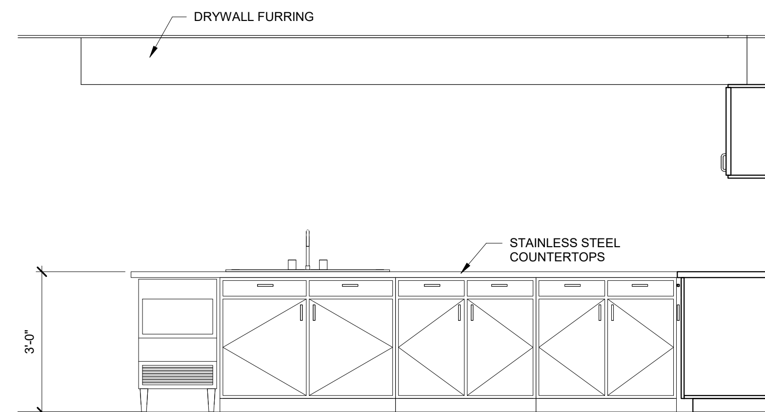
5 KITCHEN A-107 SCALE: 1/2" = 1'-0"
